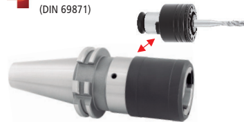
MANDRIL FLUTUANTE TROCA RÁPIDA (DIN 69871)
