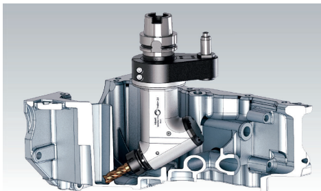
CABEÇOTE FIXO COM ÂNGULO VARIÁVEL
