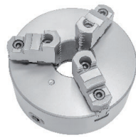
PLACA AUTOCENTRANTE COM 3 CASTANHAS REVERSÍVEIS FIXAÇÃO CAMLOCK
