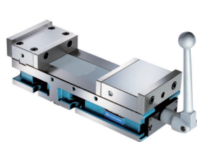
MORSA PARA CNC MULTI-POWER Modelo: HPAQ-160
